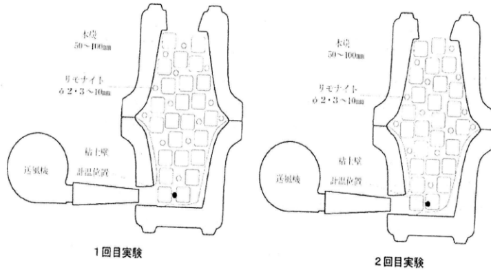
図5 リモナイトによる精錬実験炉図
